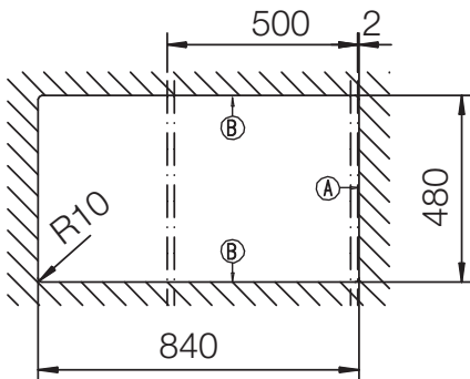
Installazione SOPRATOP
