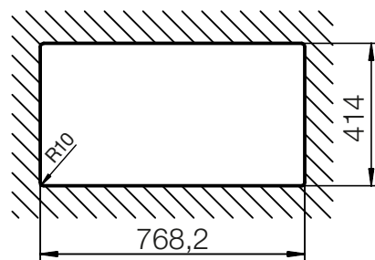
Installazione SOTTOTOP*
