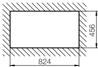
Installazione SOPRATOP
