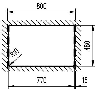
Installazione SOPRATOP
